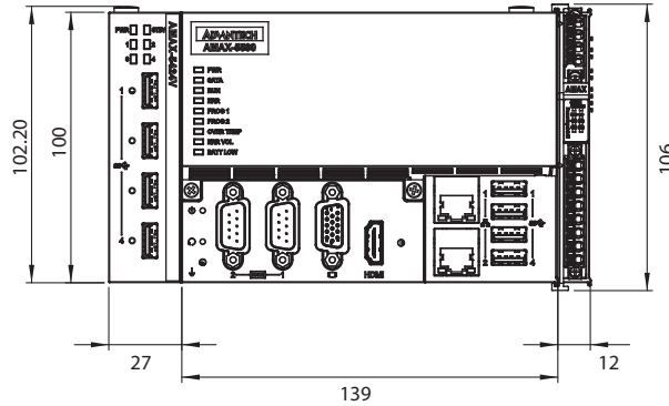
AMAX-5580 CPU Module
